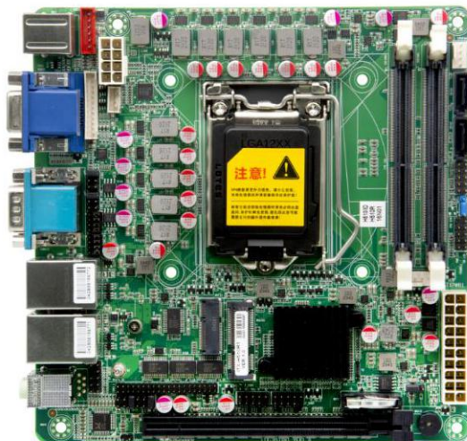
图一：ITX-H510R1 VER:1.0 正面图
