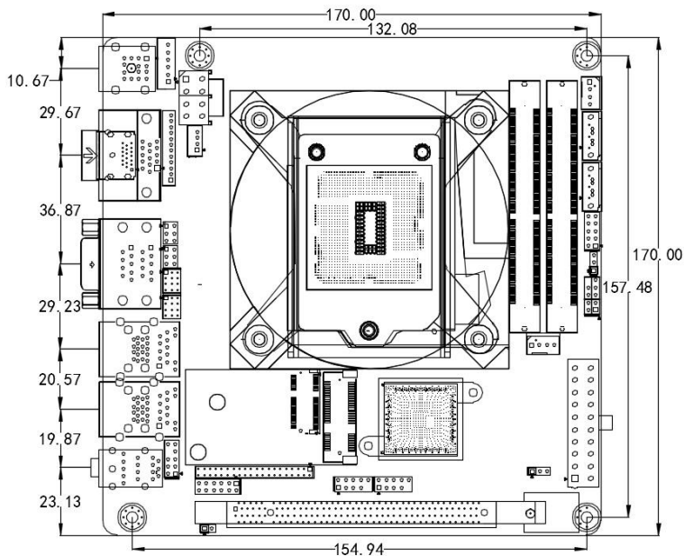
ITX-H510R1 VER:1.0 尺寸图
