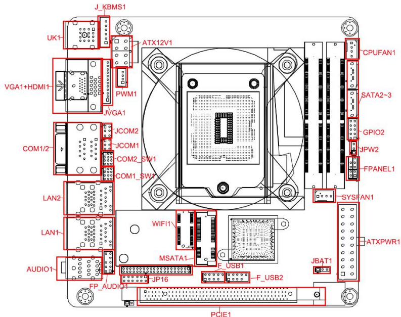
ITX-H510R1 VER:1.0 接口位置图
